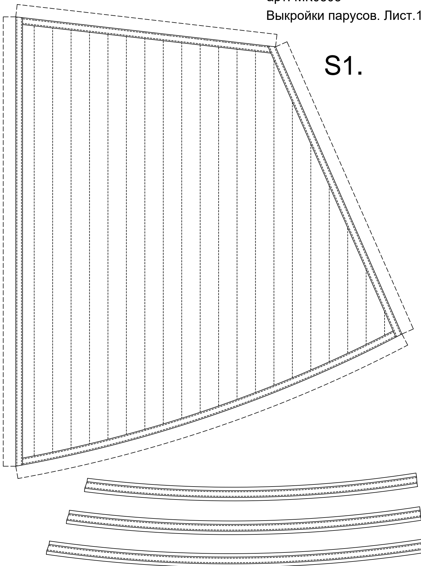
Выкройка паруса Грот S1.
